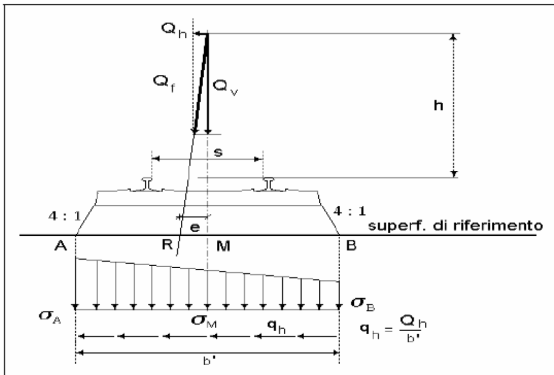
Figura 6.3.5 - Distribuzione trasversale in rettilineo delle azioni per mezzo delle traverse e del ballast
