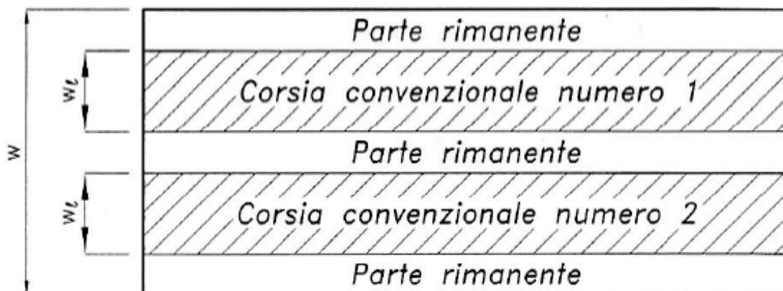
Figura 6.2.1 - Esempio di numerazione delle corsie
