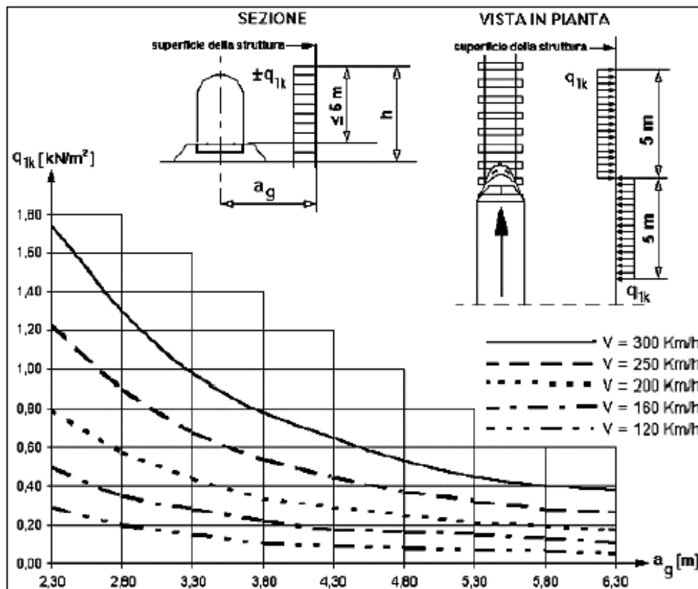
Figura 6.3.10 - Valori caratteristici delle azioni q_{1k} per superfici verticali parallele al binario
