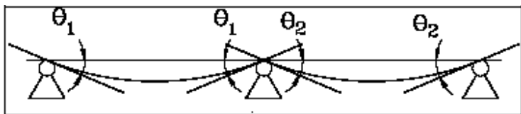
Figura 6.3.19 - Rotazioni angolari d'estremità
