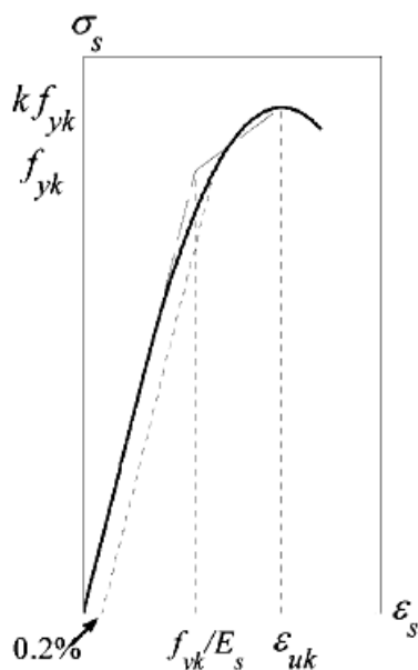
Figura 5.1.4. - Diagramma tensione/deformazione per acciaio a snervamento non definito (linea continuo) e relativo diagramma caratteristico (linea tratteggiata)
