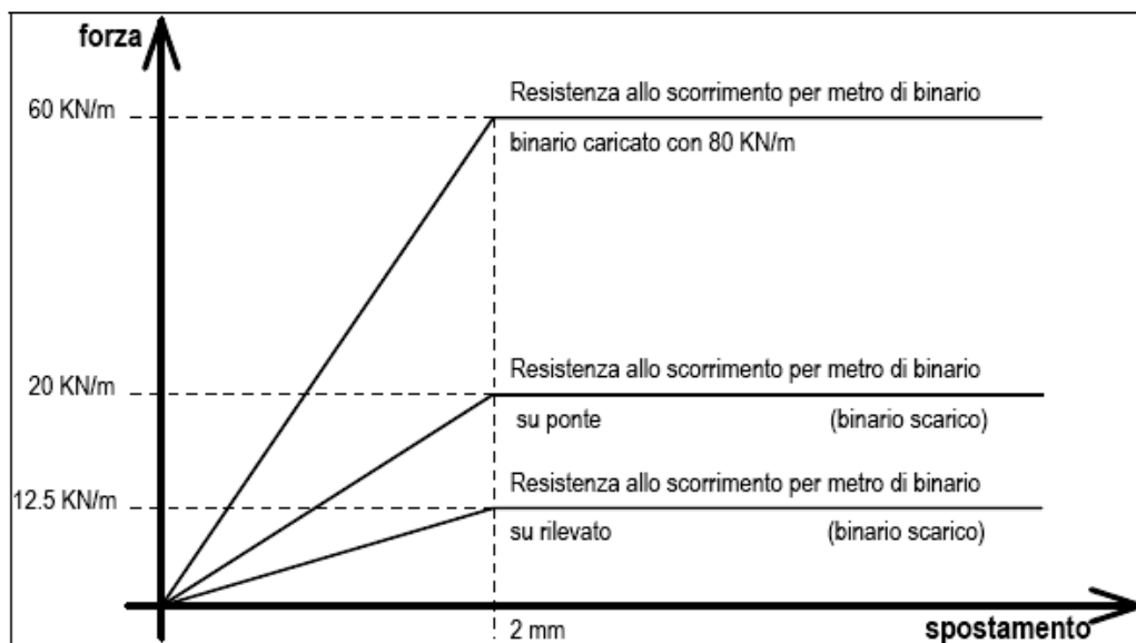
Figura 6.3.9a - Legame forza-spostamento del ballast in direzione longitudinale
