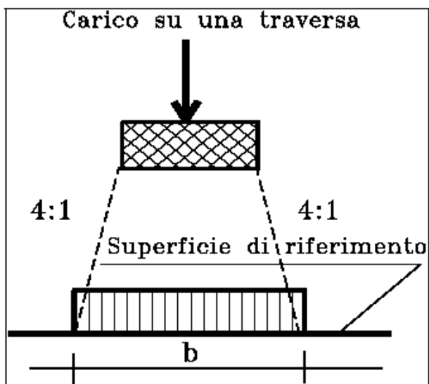
Figura 6.3.4 - Distribuzione longitudinale dei carichi attraverso il ballast
