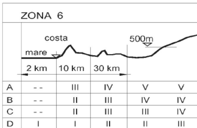
Figura 3.3.3 - Definizione delle categorie di esposizione I, II, III, IV e V, in funzione delle regioni individuate nella macrozonazione
