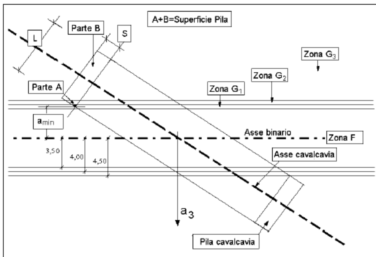
Figura 6.3.16 - Zone di rispetto orizzontali
