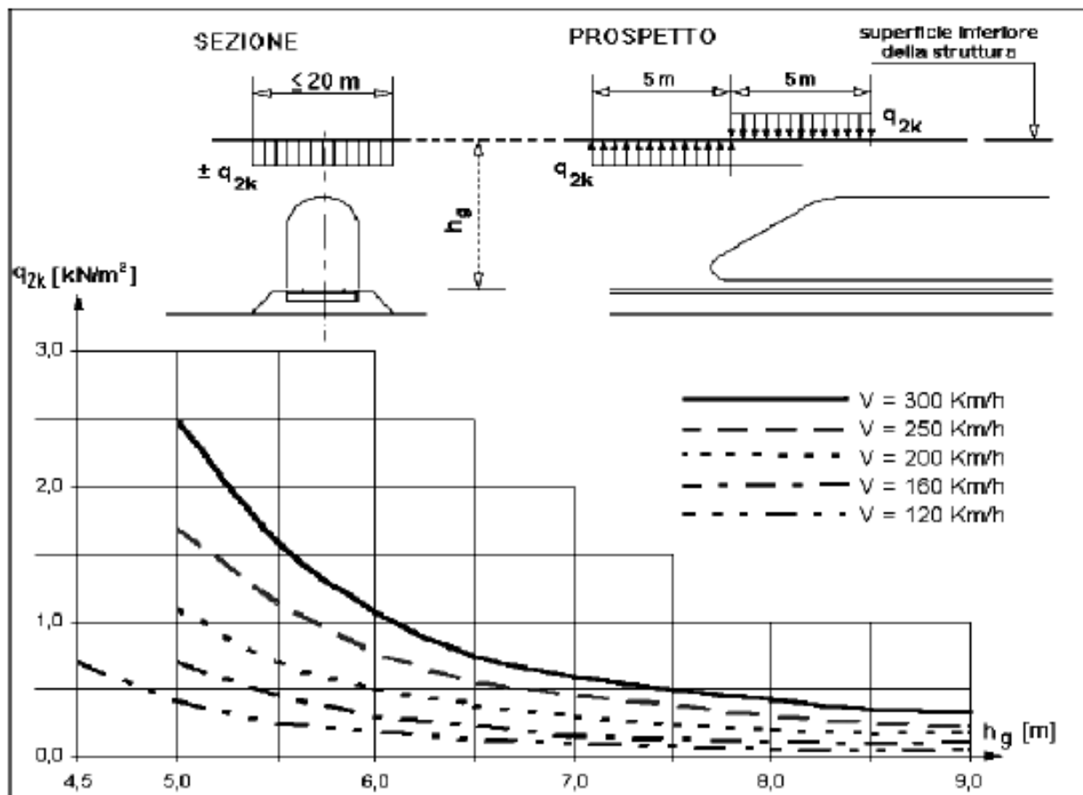
Figura 6.3.11 - Valori caratteristici delle azioni q_{2k} per superfici orizzontali al di sopra del binario
