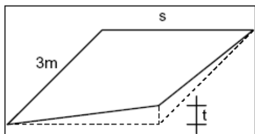
Figura 6.3.18 - Sghembo ammissibile
