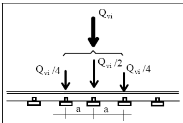
Figura 6.3.3 - Distribuzione longitudinale dei carichi assiali
