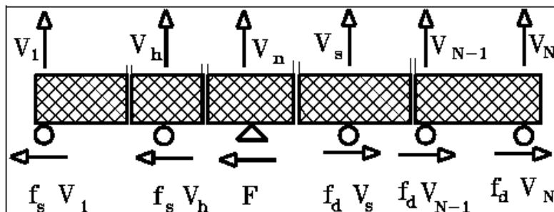
Figura 6.3.17 - Resistenze parassite nei vincoli nel caso di travi continue
