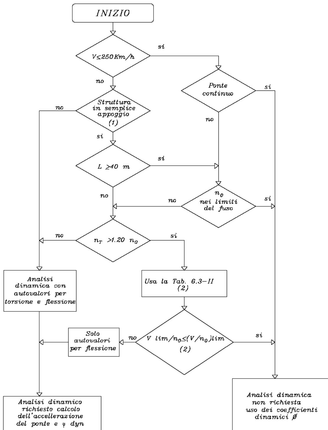
Figura 6.3.8 - Diagramma di flusso
