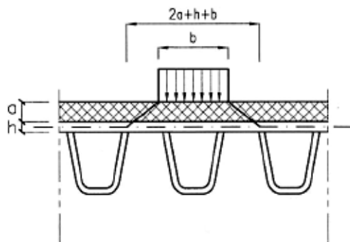
Figura 6.2.3b - Diffusione dei carichi concentrati attraverso fa pavimentazione e gli impalcati a piastra
