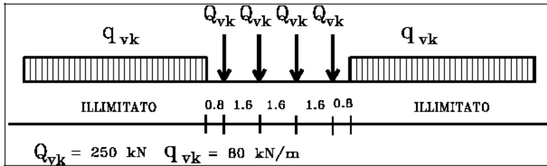
Figura 6.3.1 - Treno di carico LM 71
