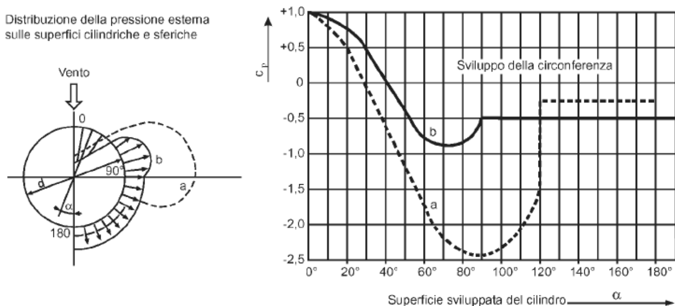
Figura 3.3.12 - Coefficienti di pressione esterna delle superfici cilindriche e sferiche: curva (a) per superfici lisce (metalli, intonaco liscio); curva (b) per superfici ruvide (muratura con giunti di malta, intonaco rustico)
