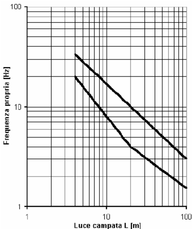
Figura 6.3.7 - Limiti delle frequenze proprie in funzione della luce
