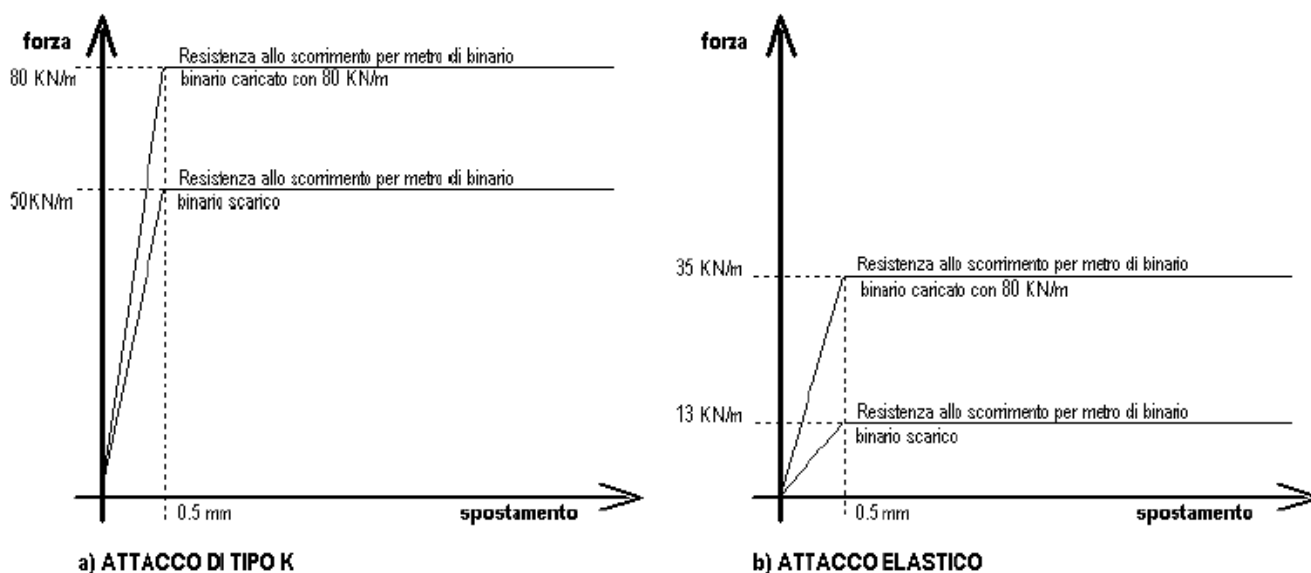
Figura 6.3.9b - Resistenza allo scorrimento nel caso di posa diretta con attacco indiretto di tipo tradizionale e con attacco elastico con interasse nominale delle traverse di 0,60 m.
