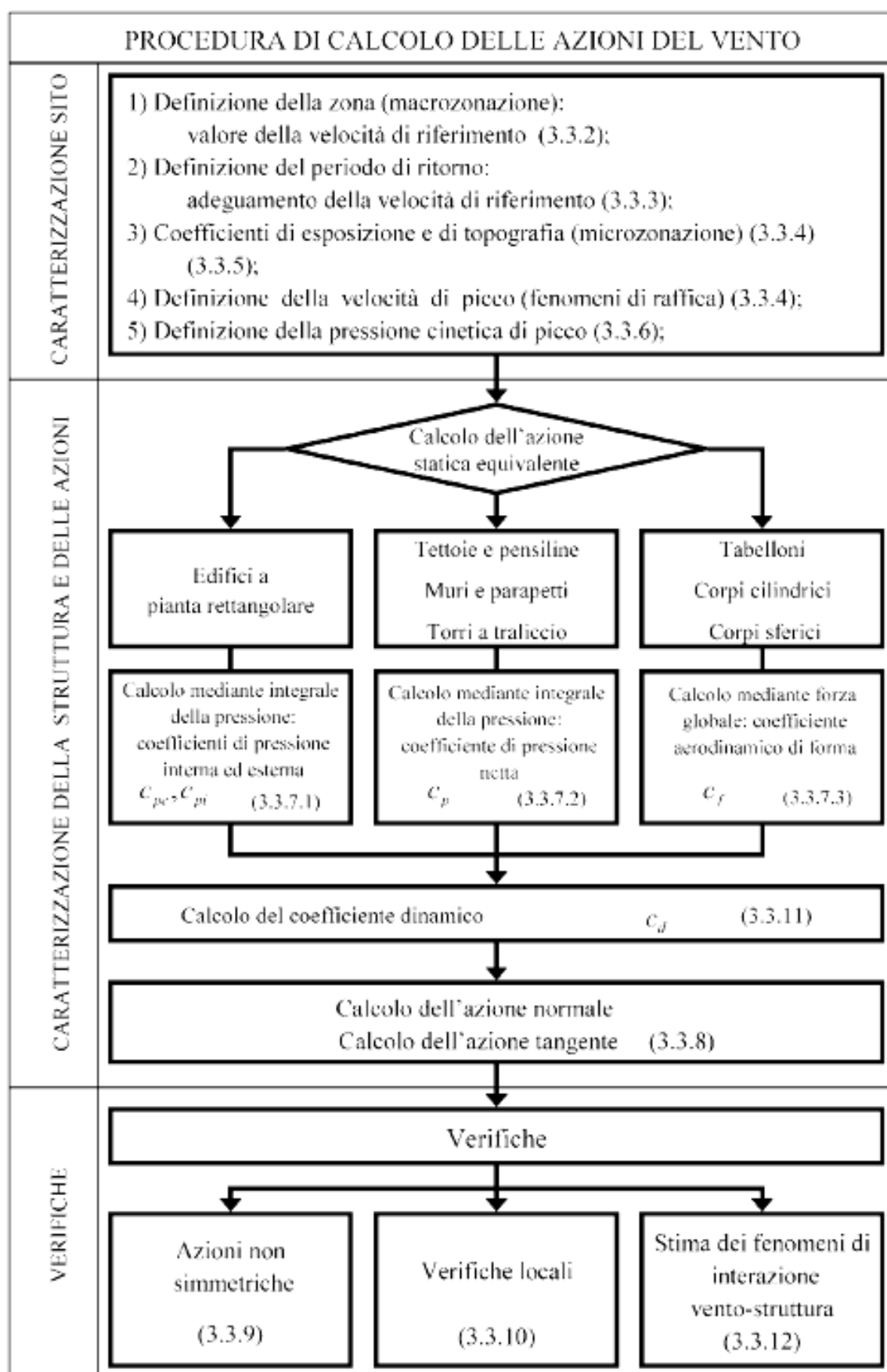
Schema 3.3.1 - Valutazione dell'azione del vento
