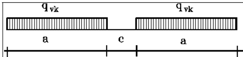
Figura 6.3.2 - Treno di carico SW
