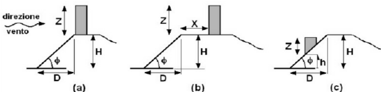
Figura 3.3.5 - Schemi di colline e pendii isolati
