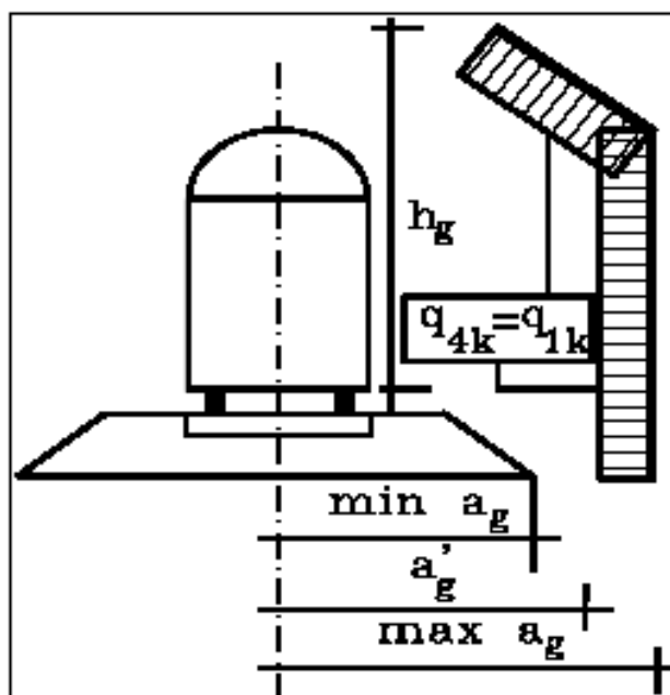
Figura 6.3.13 - Definizione della distanza \max a_g e \min a_g dal centro del binario
