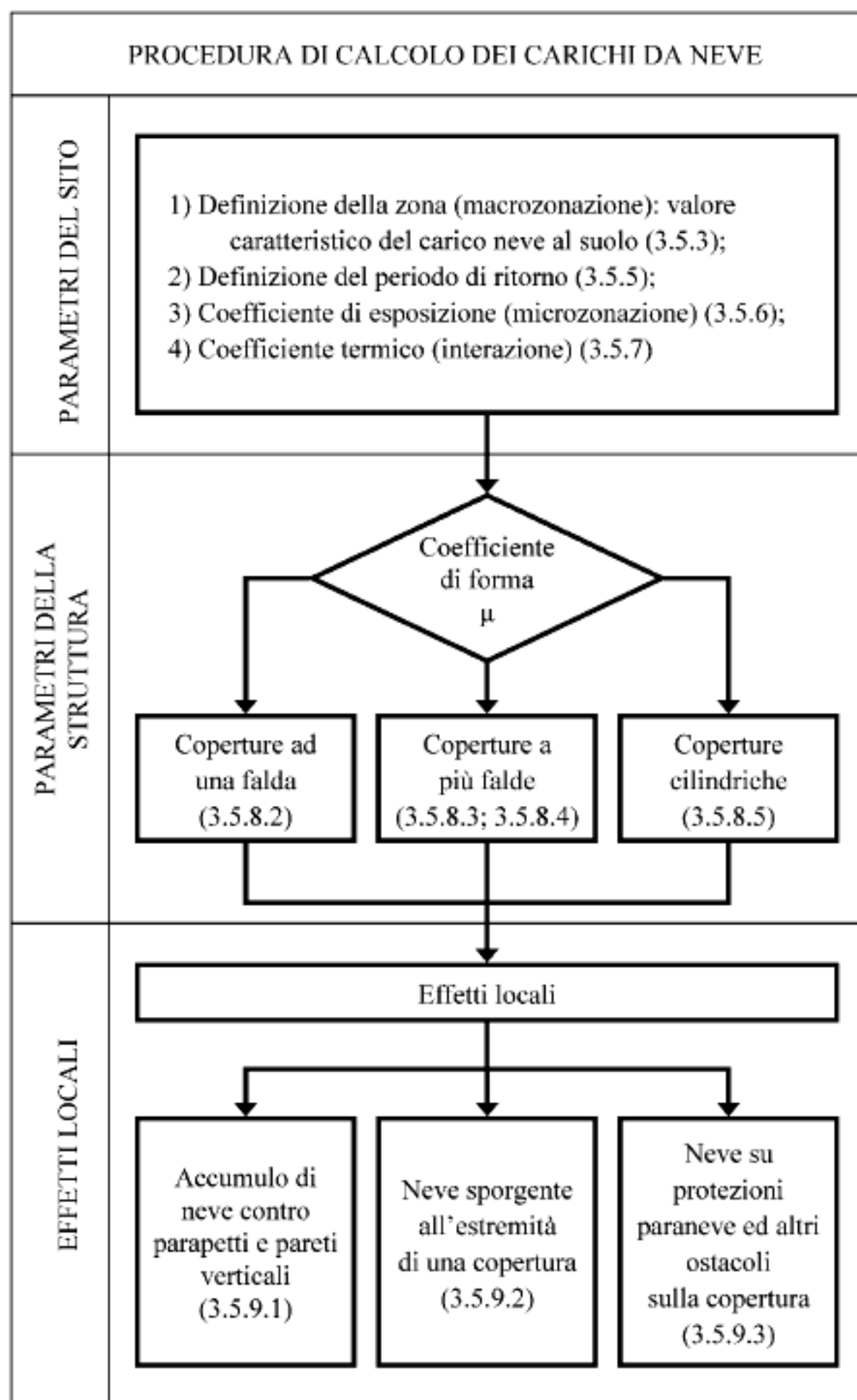
Schema 3.5.1 - Valutazione dell'azione da neve
