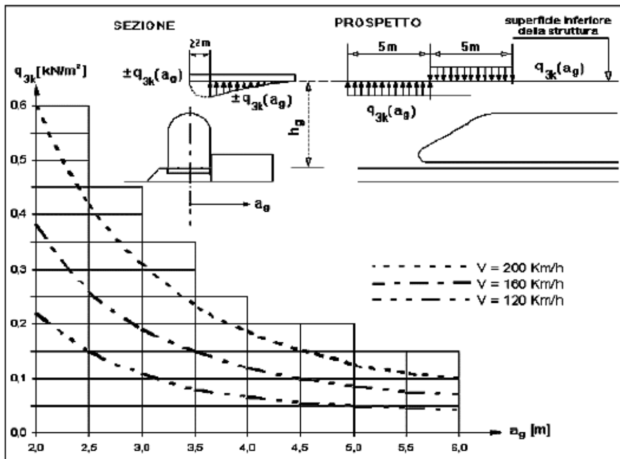
Figura 6.3.12 - Valori caratteristici delle azioni q_{3k} per superfici orizzontali adiacenti il binario
