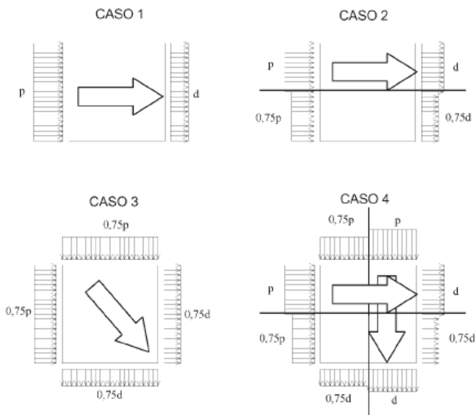
Figura 3.3.9 - Distribuzioni non simmetriche delle pressioni
