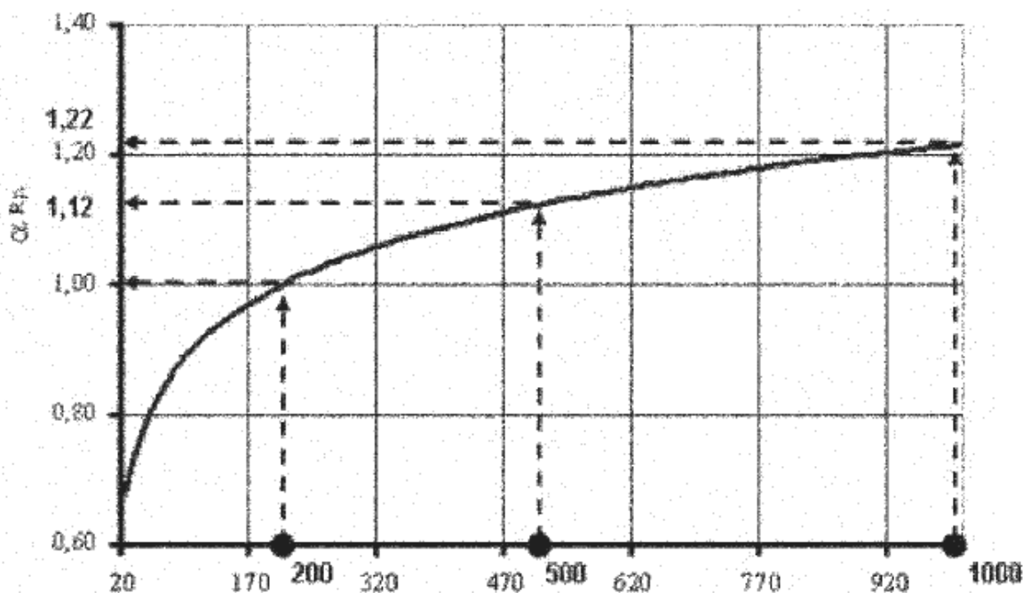
Figura 3.5.2 - Valori del coefficiente a_{Rn} = q_{ref}/q_{sk} in funzione del periodo di ritorno T_r
