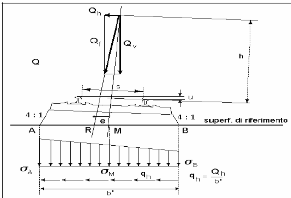
Figura 6.3.6 - Distribuzione trasversale in curva delle azioni per mezzo delle traverse e dei ballast
